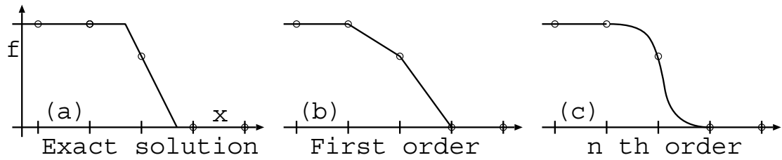
図 6: 格子間の補間の例．線形補間 (b) を使った場合，プロファイルが大きく崩れる． n ( n > 1 ) 次の補間を使う場合 (c)，線形補間 (b) よりも，厳密解 (a) に近づくことが期待される．
