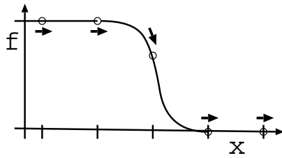
図 8: CIP 法の意味 .
